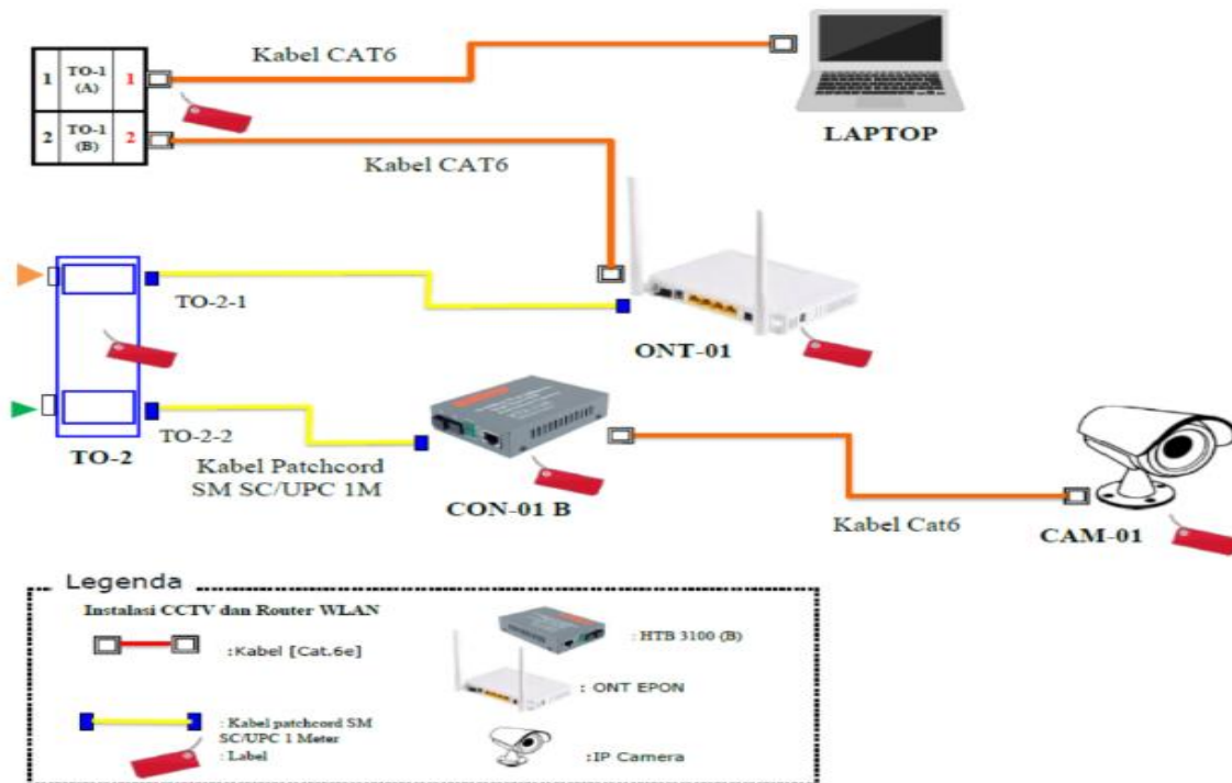
Skema Modul 1.2 Konfigurasi Network Equipment
